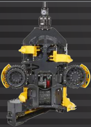
PONSSE H6
